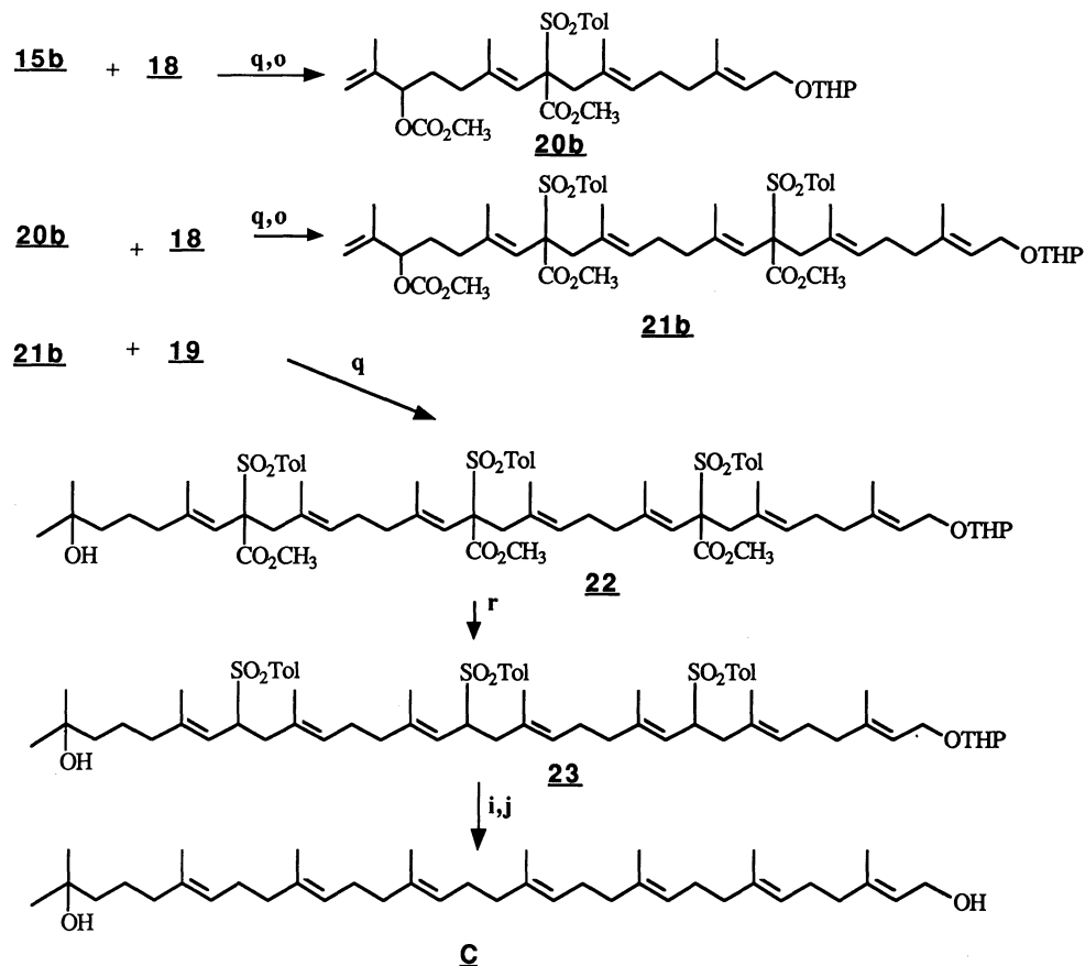
Scheme 5. i: Na/Hg, Na 2 HPO 4 /MeOH; j: TsOH/EtOH; o: ClCO 2 Me, Py/Tol; q: (Ph 3 P) 4 Pd/Et 2 O; r: PATP, CsCO 3 /DMF.
